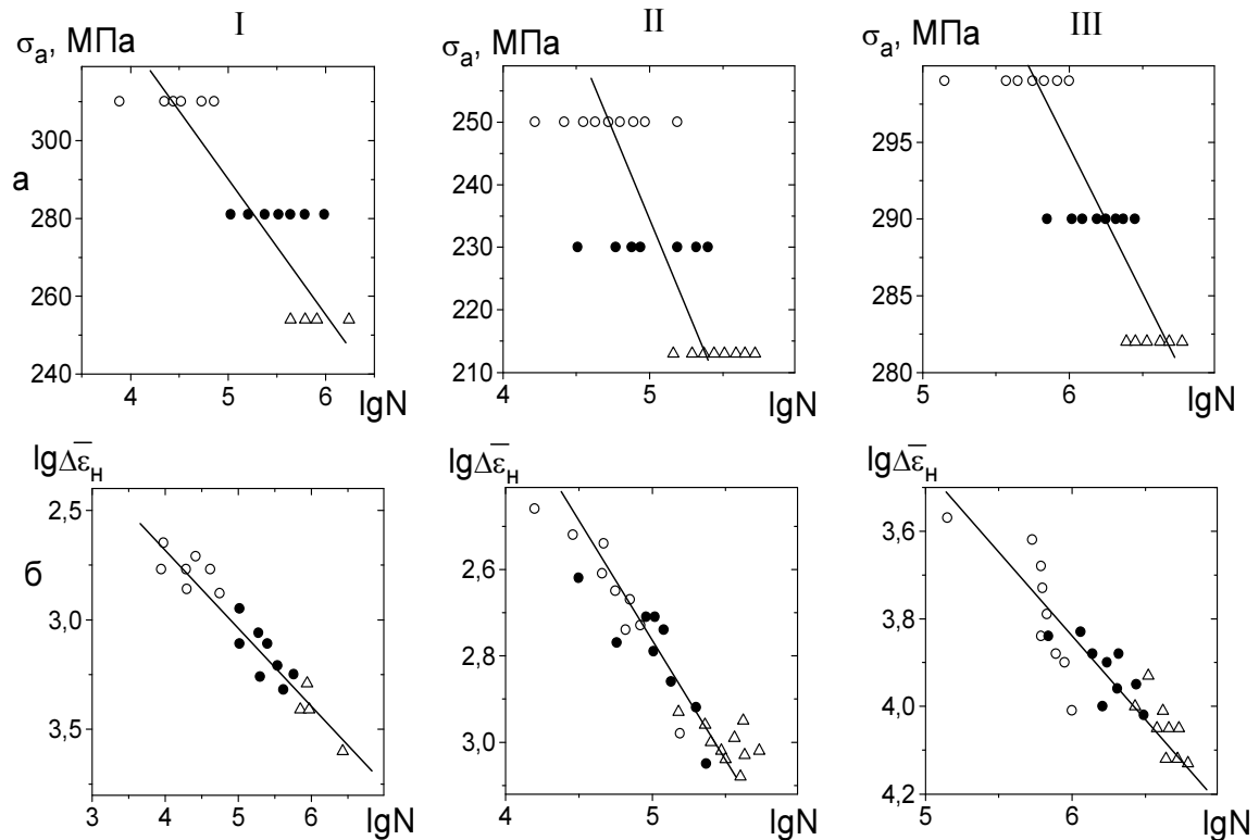
Рисунок 3. Криві втоми сталей 15Г2АФДпс (I), 45 (II) і 1Х13 (III) в координатах \sigma_a - \lg N (а) і \lg \Delta \bar{\epsilon}_n - \lg N_p (б)
